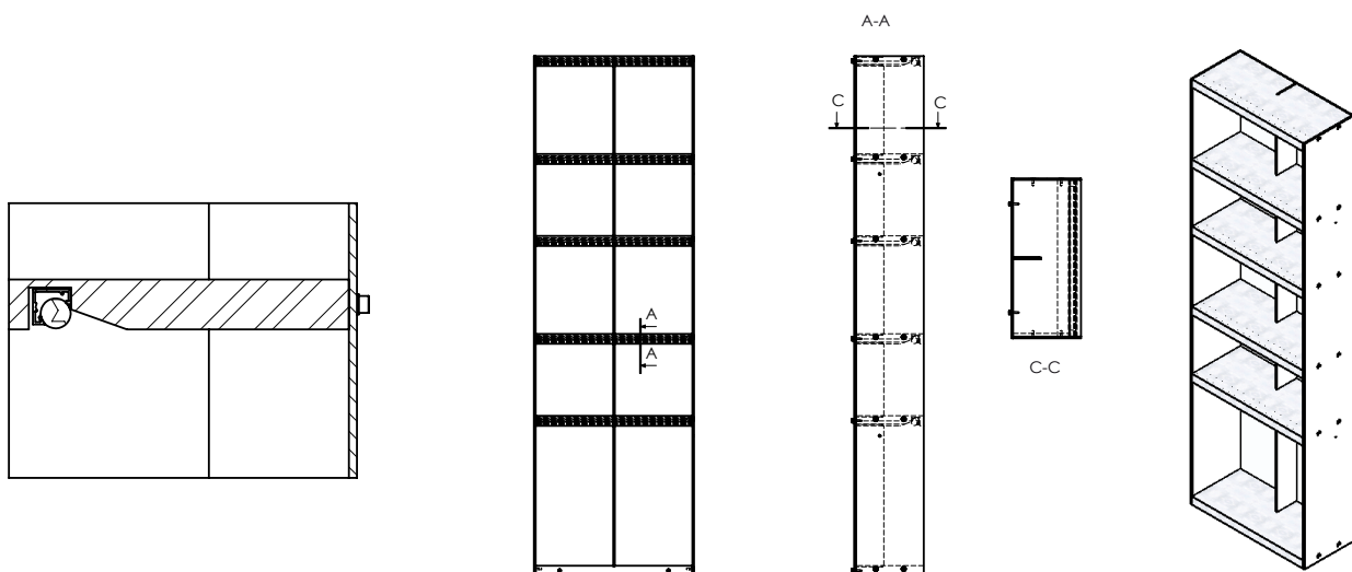
Konstruktionsansichten der Metallvittrinen
