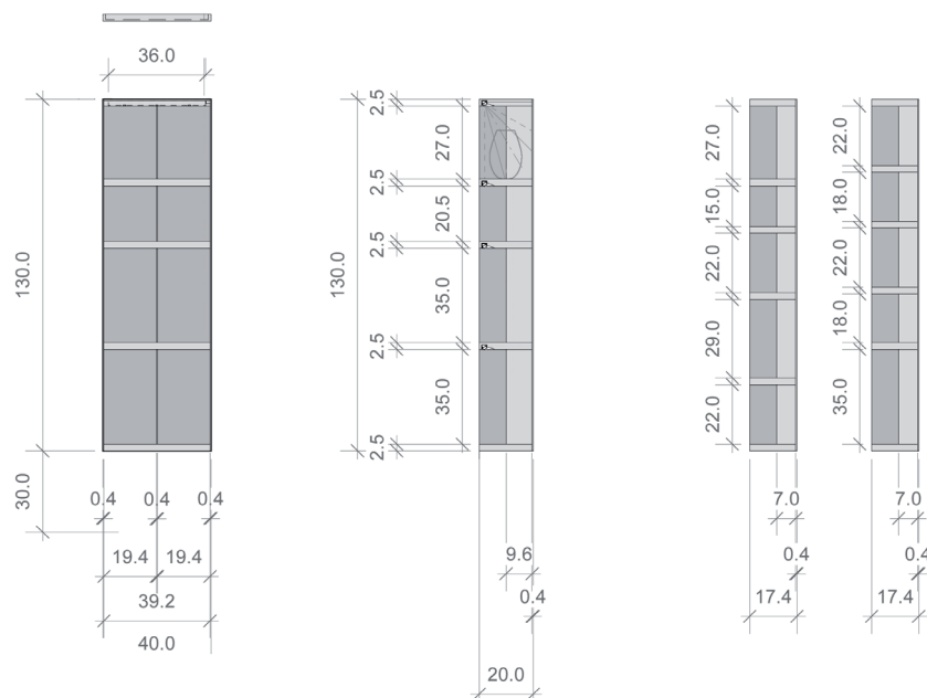
Frontal- und Seitenansicht der drei Nischentypen
